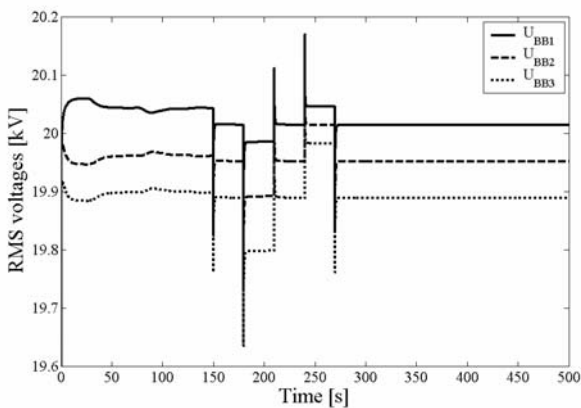
Fig. 23. Bus bar voltages.
