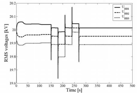
Fig. 17. Bus bar voltages.
